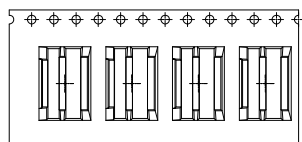
产品入载带示意图
